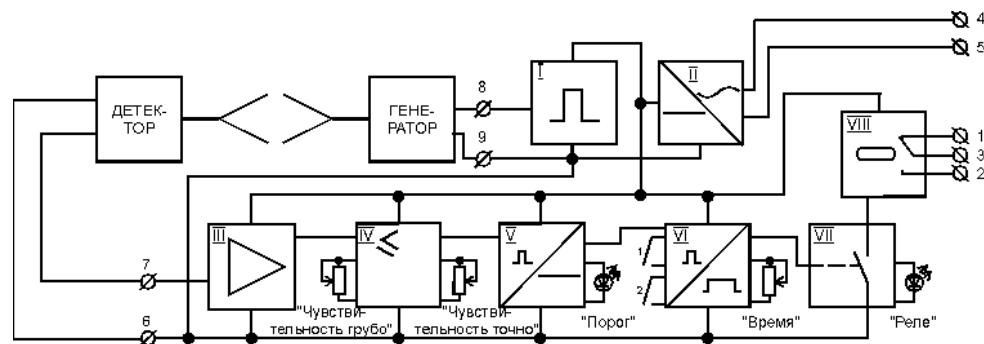
Рис. 2. Структурная схема датчиков уровня серии PCY-500.
